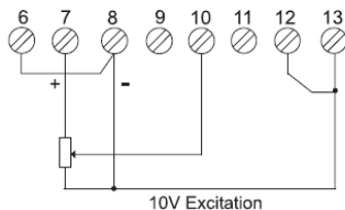
Potentiometer
